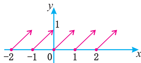
График функции y = \{x\}
