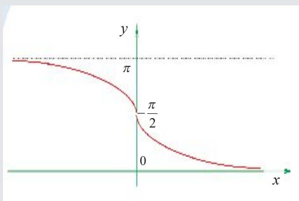
График функции y = \text{arccctg}x
