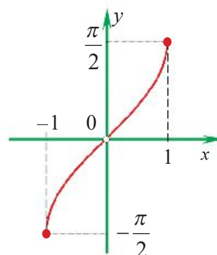
График функции y = \arcsin x
