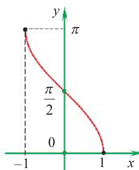
График функции y = \arccos x
