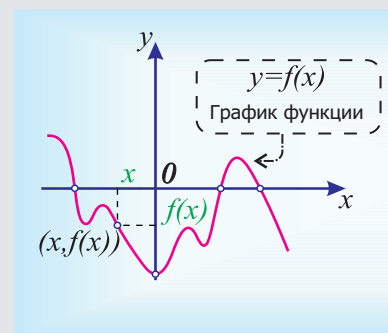
График функции f(x)
