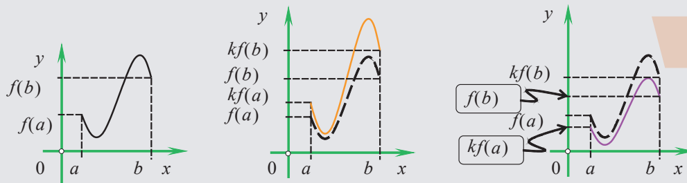
Построение графика функции y = kf(x)
