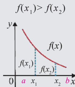
Убывающая функция
