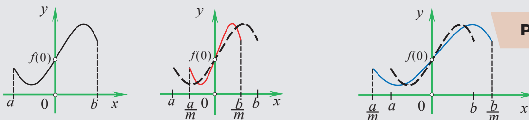
Построение графика функции y = f(mx)
