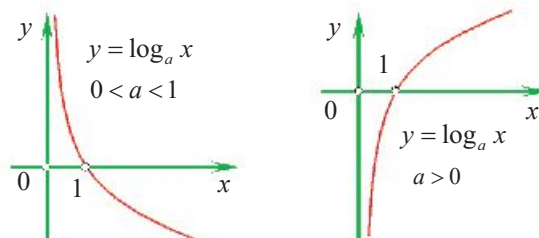
График логарифмической функции
