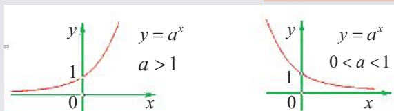
График показательной функции
