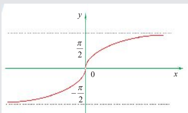
График функции y = \operatorname{arctg} x
