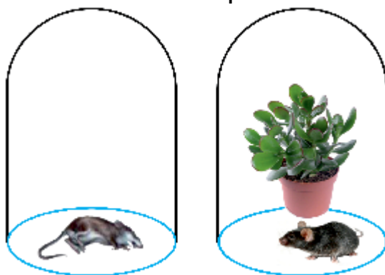
Рис. 28. Опыт Пристли
