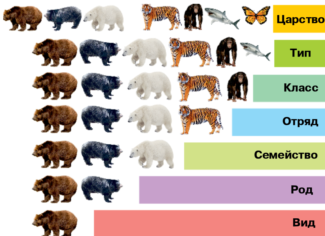
Рис. 55. Классификация животных
