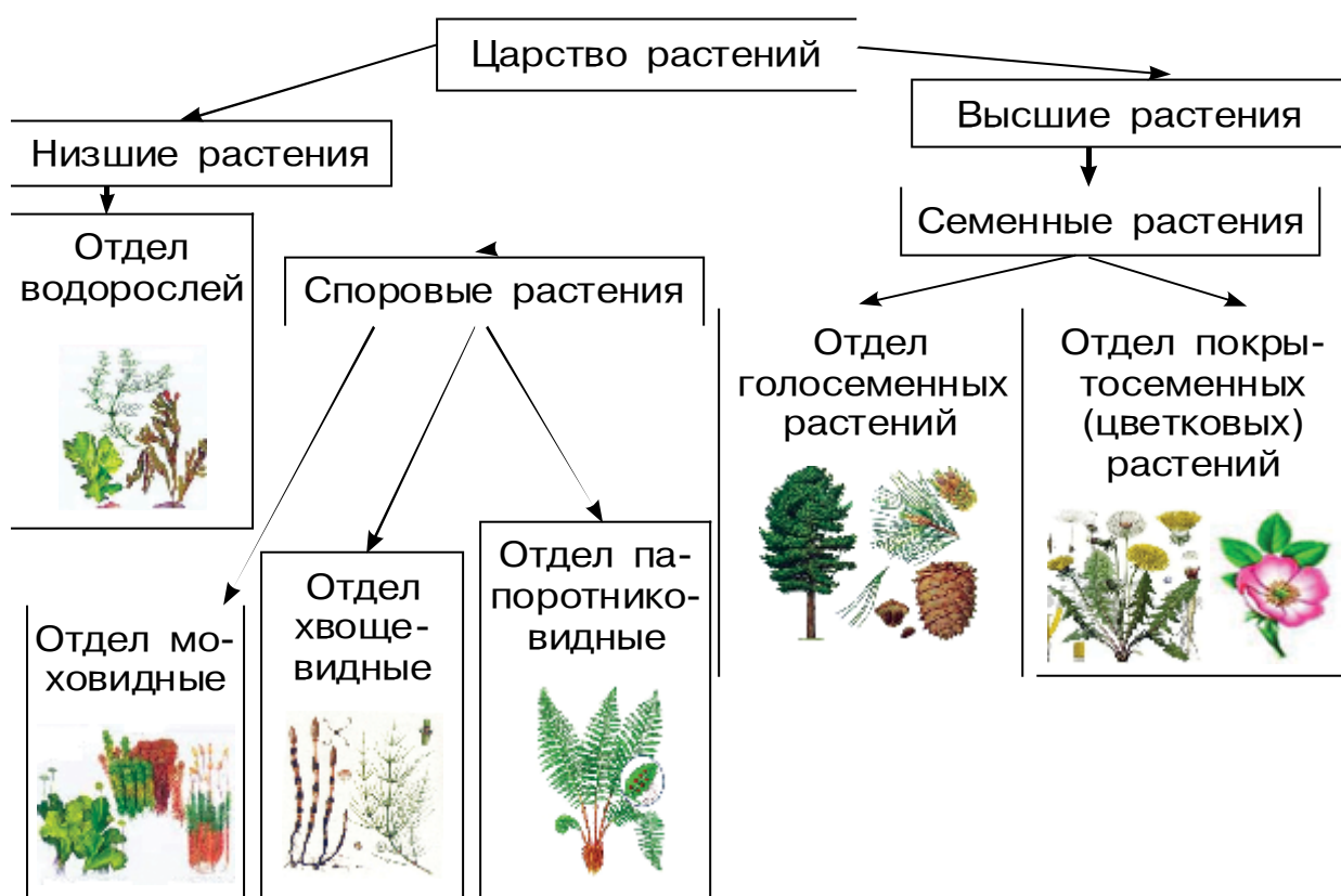
Рис. 27. Систематика растений
