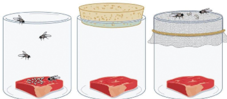
Рис. 9. Опыт Реди
