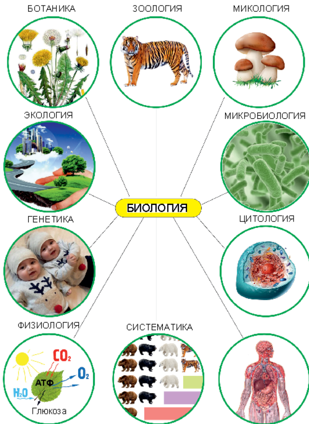
Рис. 1. Разделы биологии
