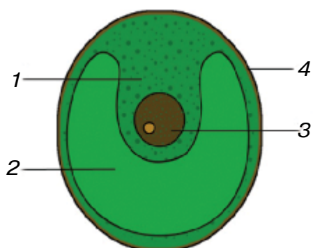
Рис. 29. Хлорелла:
