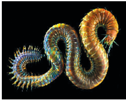
Рис. 60. Кольчатые черви:
