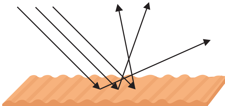
Рисунок, показывающий отражение света от шероховатой поверхности
