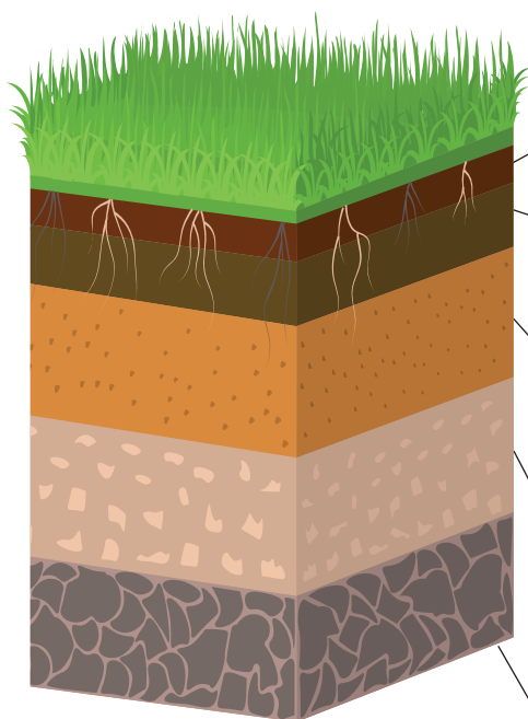
Слои почвы
