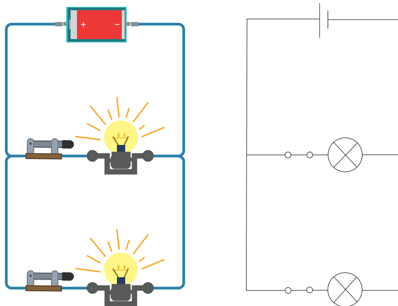
Электрическая цепь, состоящая из двух параллельно соединённых электрических ламп, ключей, и её схема
