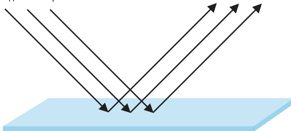
Рисунок, показывающий отражение света на плоской гладкой поверхности
