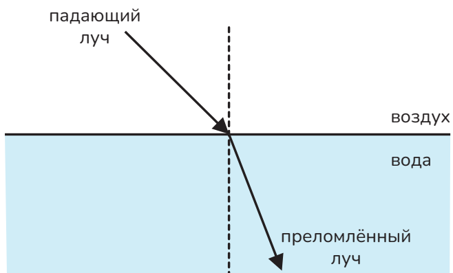
Рисунок, показывающий преломление света
