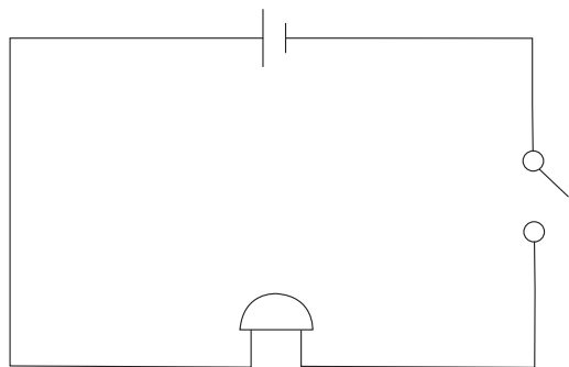
Elektr qo'ng'iroqni zanjirga ulash sxemasi
