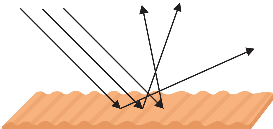
Yorug'lik nurlarining g'adir-budur sirtga qaytishini ko'rsatuvchi chizma
