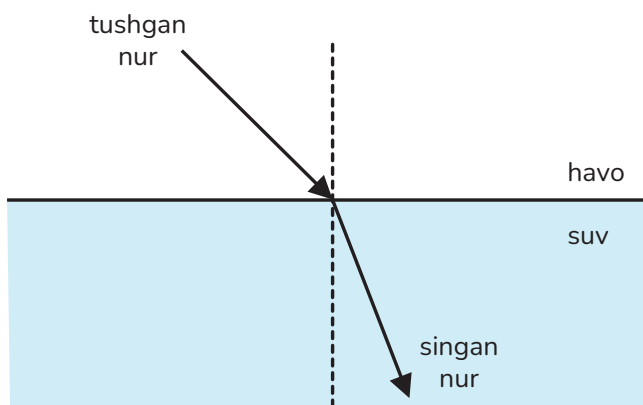
Yorug'lik nurining sinishi ko'rsatilgan chizma
