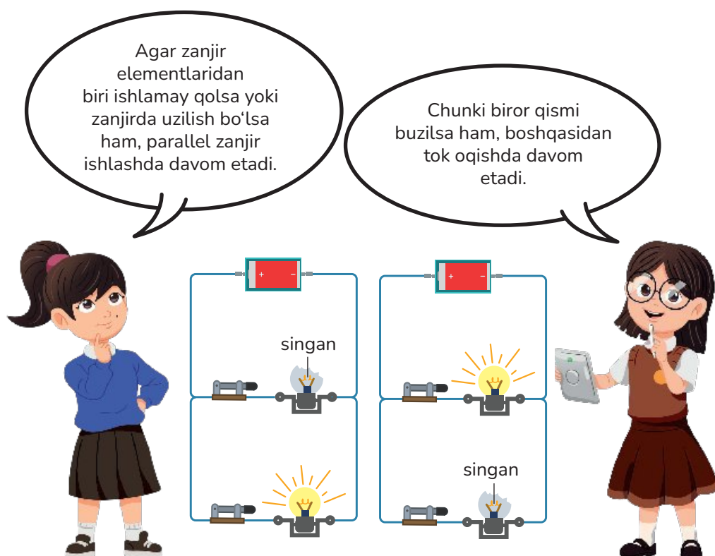
Ikkita chiroq, ikkita kalit va batareyadan iborat parallel ulangan elektr zanjir va uning sxemasi
