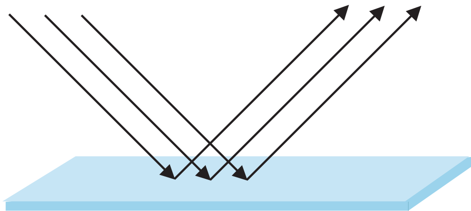
Yorug'lik nurlarining yassi silliq sirtga qaytishini ko'rsatuvchi chizma
