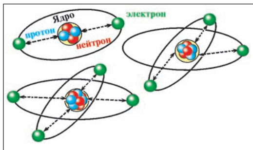
Рис.3. Строение атома
